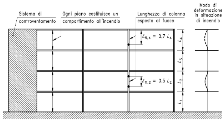
Figura 5-19 – Lunghezza libera di inflessione di colonne in caso d'incendio nel caso di telai controventati
